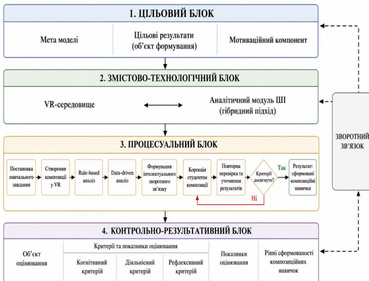
Рис. 1. Структурно-функціональна модель автоматизованого оцінювання та формування композиційних навичок у VR-середовищі на основі гібридного ШІ
