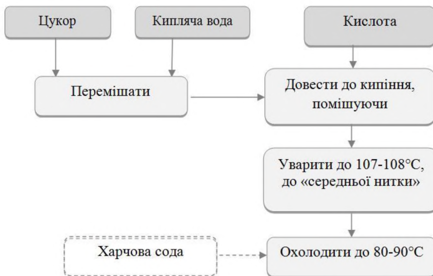
Рис. 3.2.1.3. Технологічна схема приготування інвертного сиропу
