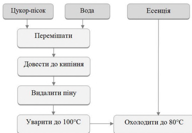
Рис. 3.2.1.2. Технологічна схема приготування сиропу для глазурування (тираажного)
