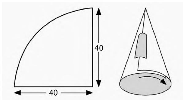
Рис. 4.6.6.2. Виготовлення конуса
