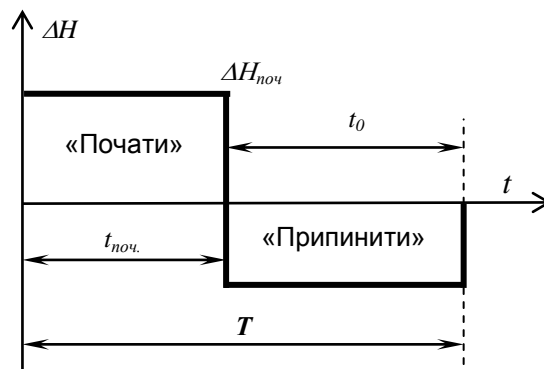
Рис. 2.3. Знакозмінна ентропія
