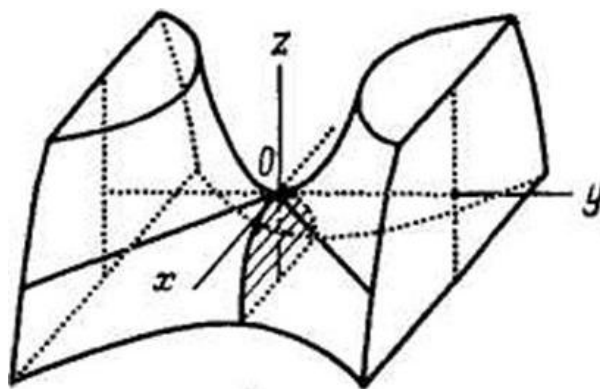
Рис. 1.13. Морсовське сідло
