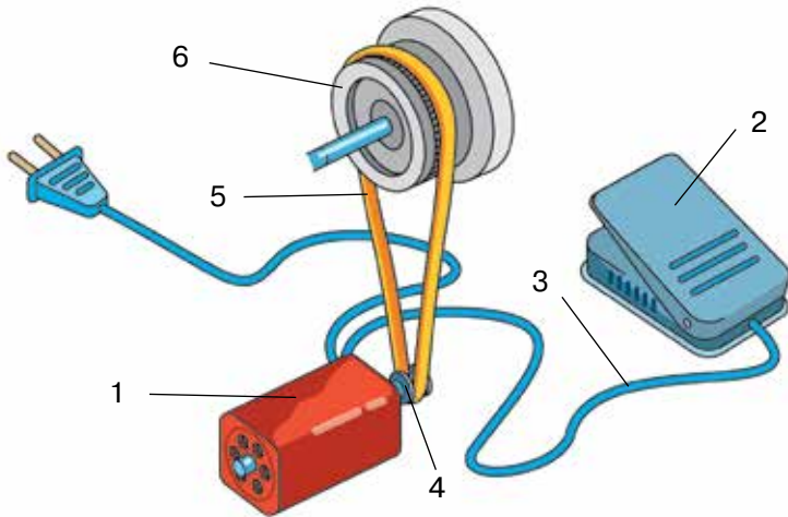
Мал. 129. Електричний привод: 1 — електродвигун; 2 — пускорегульовальна педаль; 3 — з'єднувальний шнур; 4 — шків електродвигуна; 5 — пас; 6 — шків махового колеса
