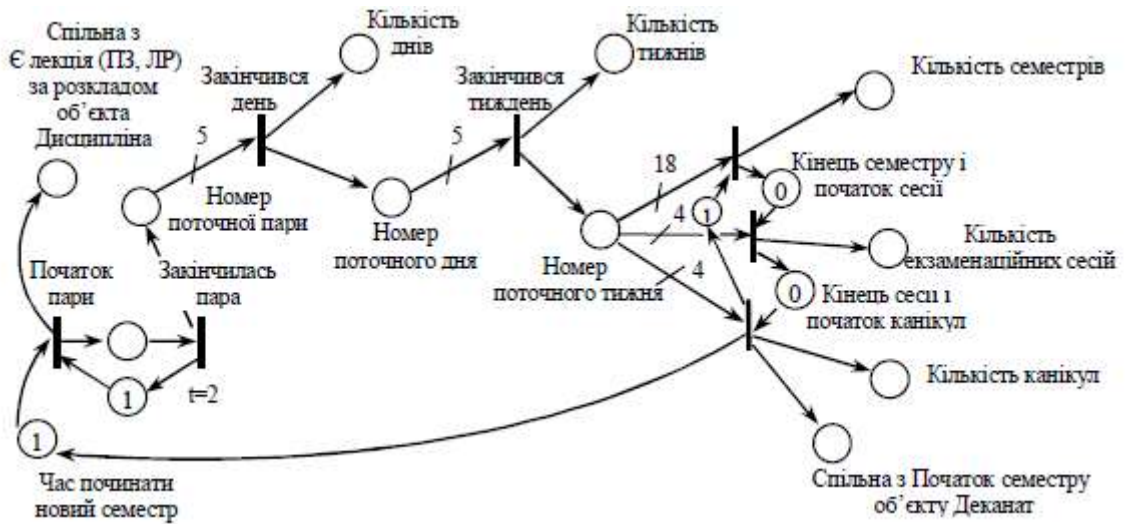
Рис. 1. Мережа Петрі об'єкта Розклад
