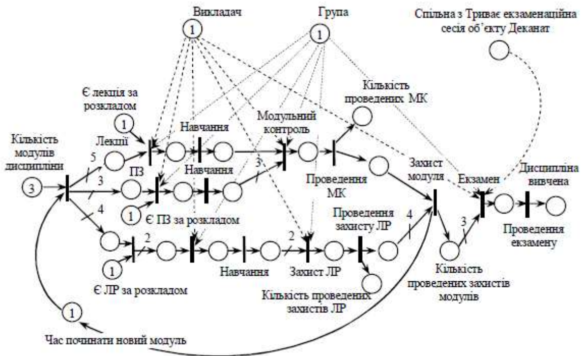
Рис. 2. Мережа Петрі об'єкта Дисципліна
