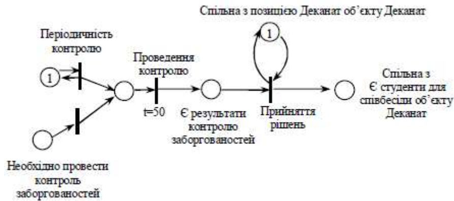
Рис. 6. Мережа Петрі об'єкта Контроль
