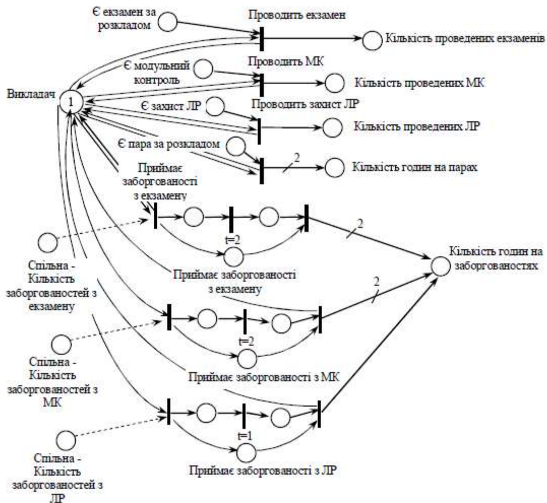
Рис. 3. Мережа Петрі об'єкта Викладач
