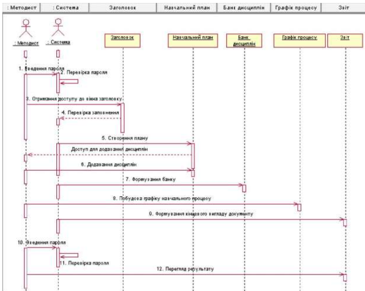
Рис. 4. Діаграма послідовності
