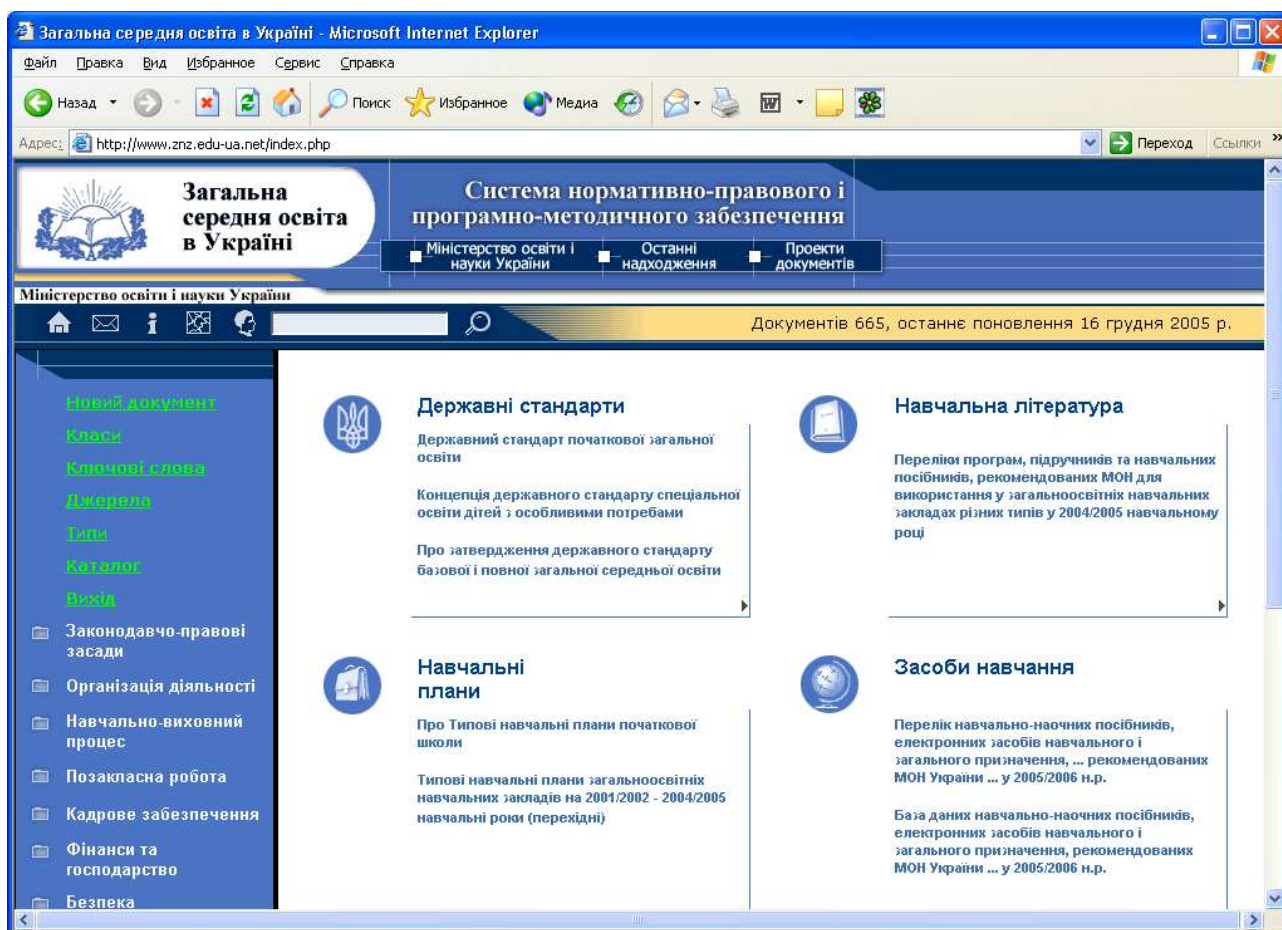
Рис. 3. АРМ контент-адміністратора
