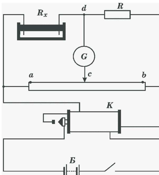
Рис. 1. Місткова схема для визначення питомої електропровідності ґрунту
