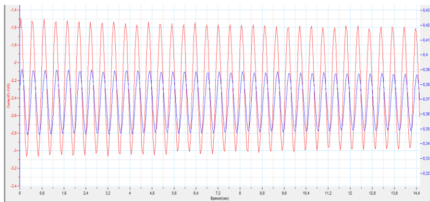
Рис. 3 Графік залежності координати і сили від часу
