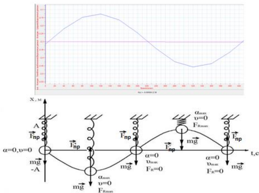
Рис. 9 Графік залежності амплітуди коливань від часу
