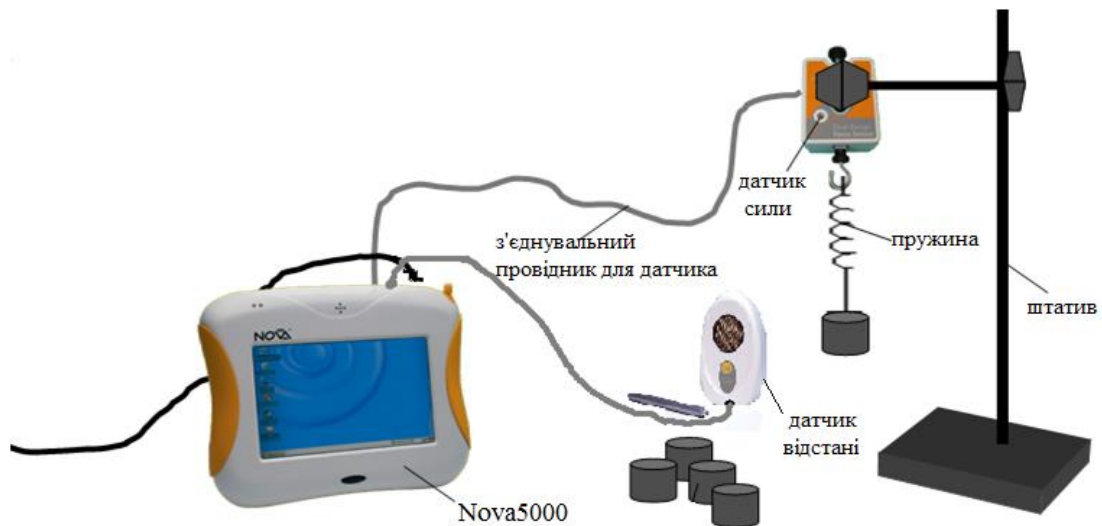
Рис.2 Схема експериментальної установки
