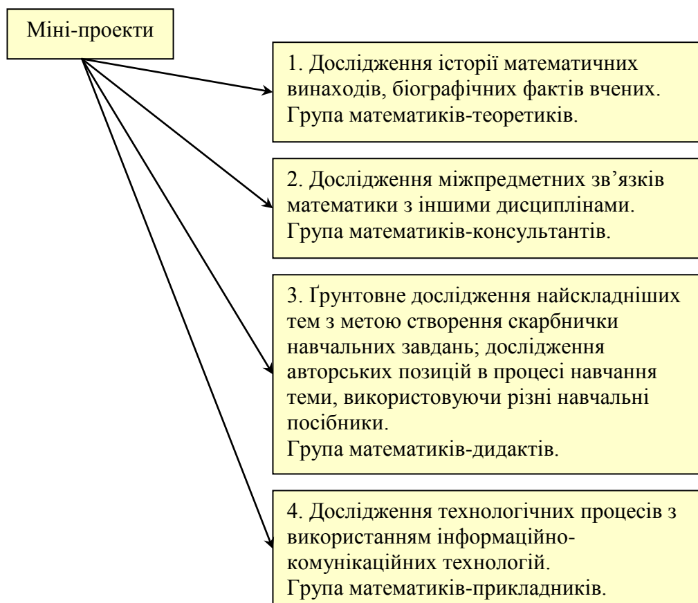
Рис. 6. Структура міні-проектів
