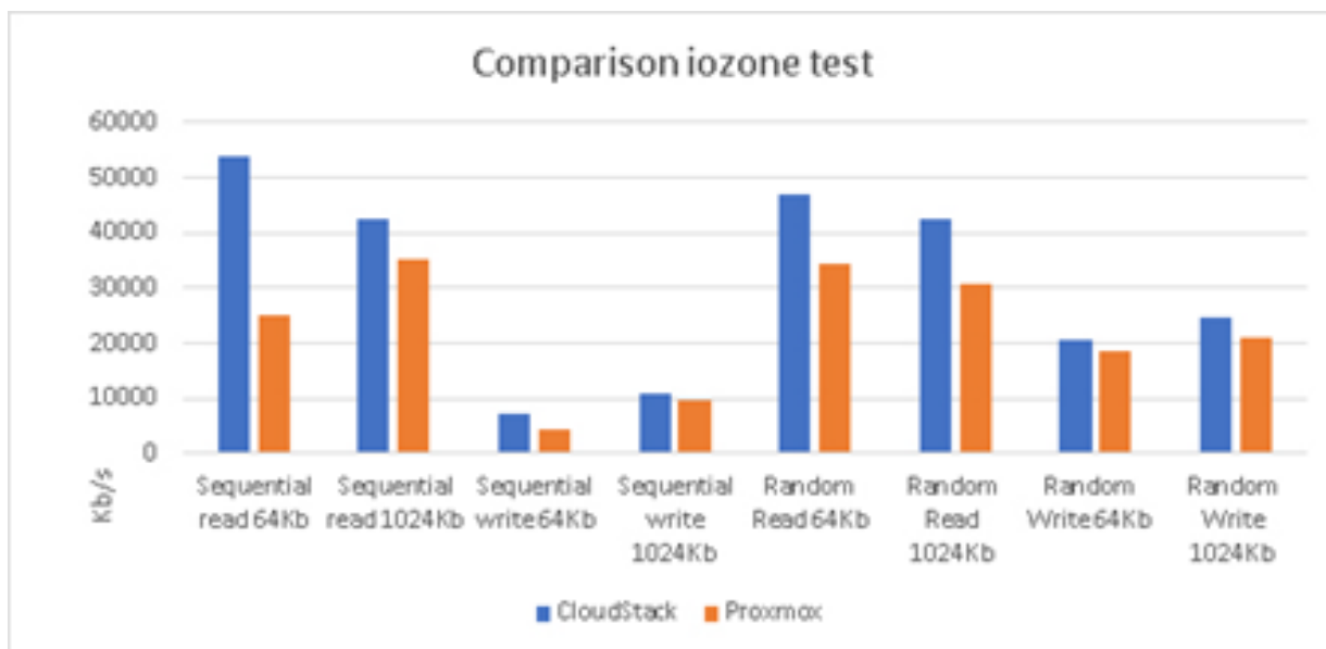
Рис. 5.1.1. Порівняння результатів тесту iозone
