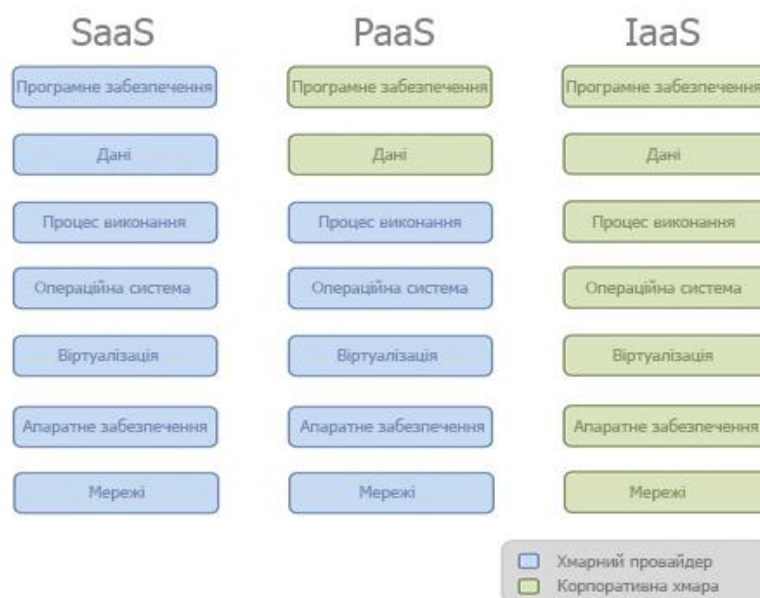
Рис. 2.3.4. Діаграма відповідності сервісних та моделей розгортання ХОСН (на основі [218] та [377])
