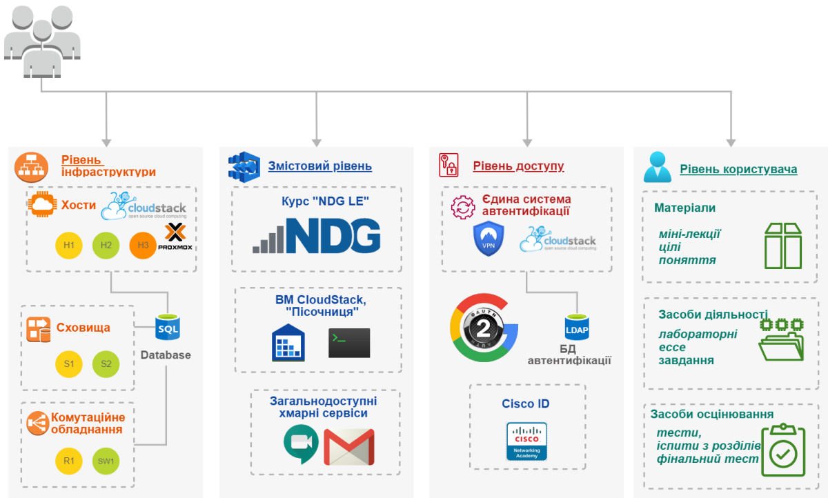
Рис. 4.1.1. Архітектура хмарної лабораторії CL-OS
