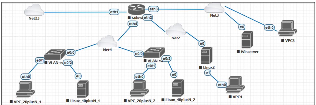
Рис.4.3.1. Топологія мережі з використанням технології VLAN
