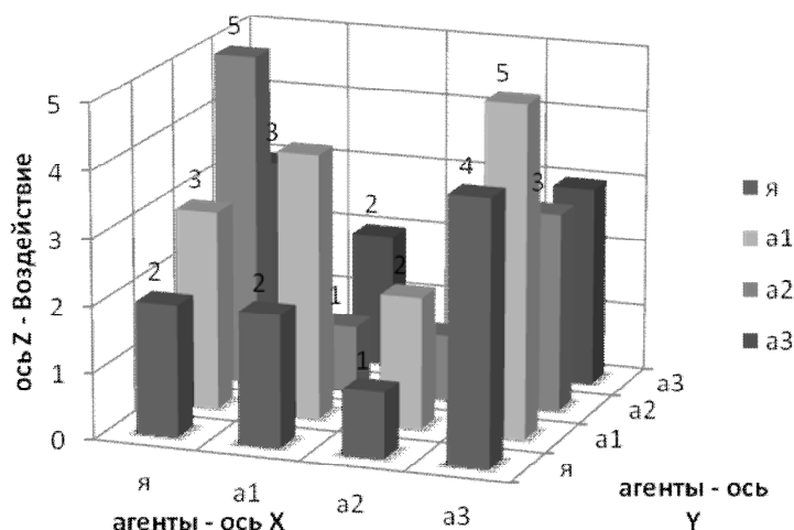
Рис. 1 Двумерная СПД с переменными: агенты и воздействия
