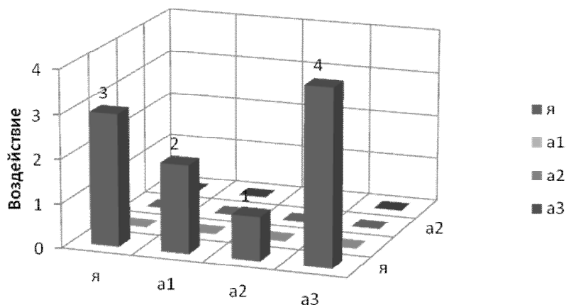
Рис. 2. Агенты я , а1 , а2 , а3 с различной степенью влияния
