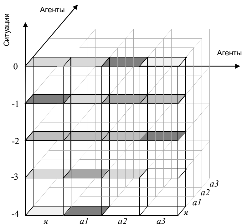
Рис. 3. Трёхмерная СПД с возможными вариантами динамики влиятельности агентов в интракультуре лица
