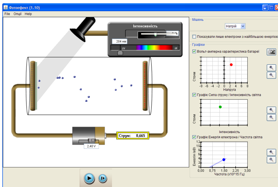
Рис. 1. Модель для дослідження явища фотоефекту
