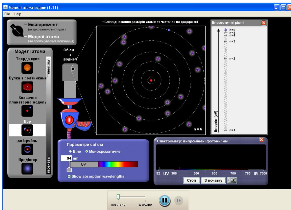
Рис. 2. Моделі атома водню
