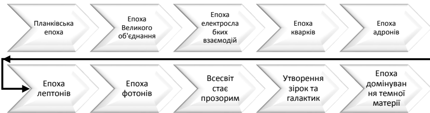
Рис. 4. Періоди розвитку Всесвіту
