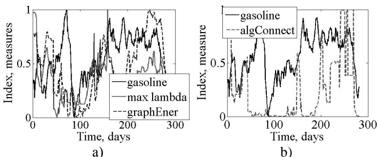
Рис. 14. Порівняльна динаміка спотових цін на бензин з максимальним власним значенням та енергією графу (a) і мірою алгебраїчної зв'язності (b), розрахованих за методом CRP
